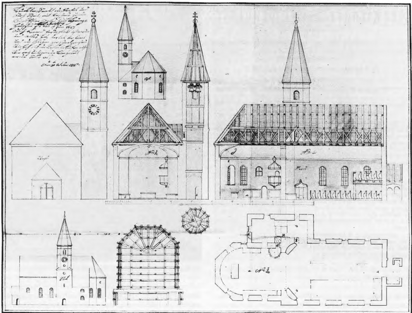
Bauplan zum Wiederaufbau der Kirche von Paunzhausen.
