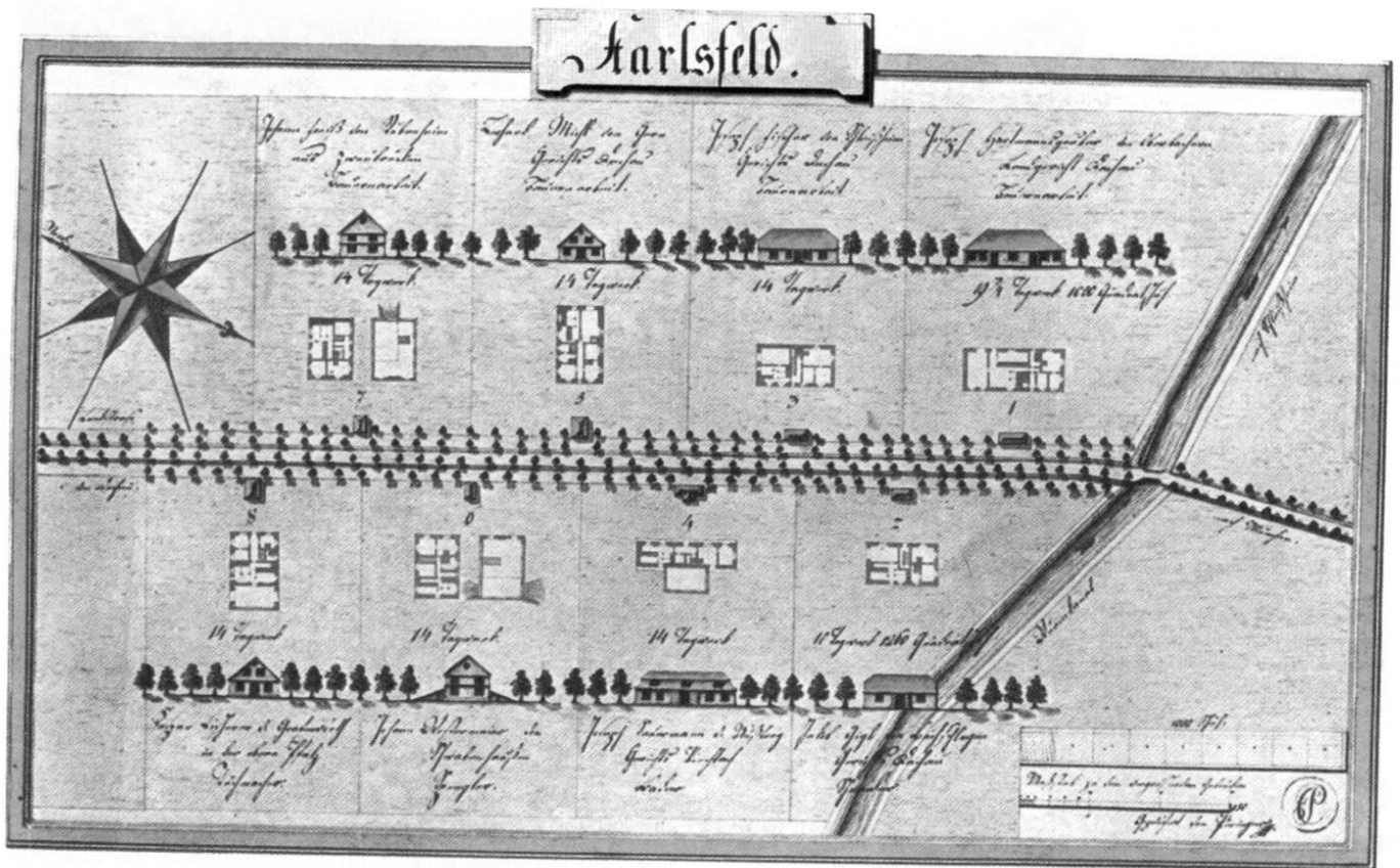
Lageplan, Grundriss und Ansicht der ersten Siedlungshäuser von Karlsfeld. Kolorierte Handzeichnung 1802.
