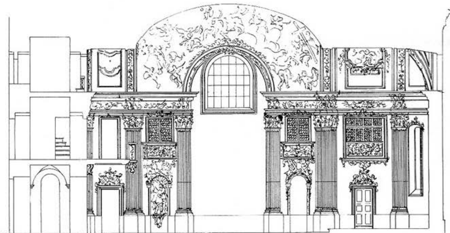
Hofmarkkirche Schönbrunn, Innenlängsschnitt.
