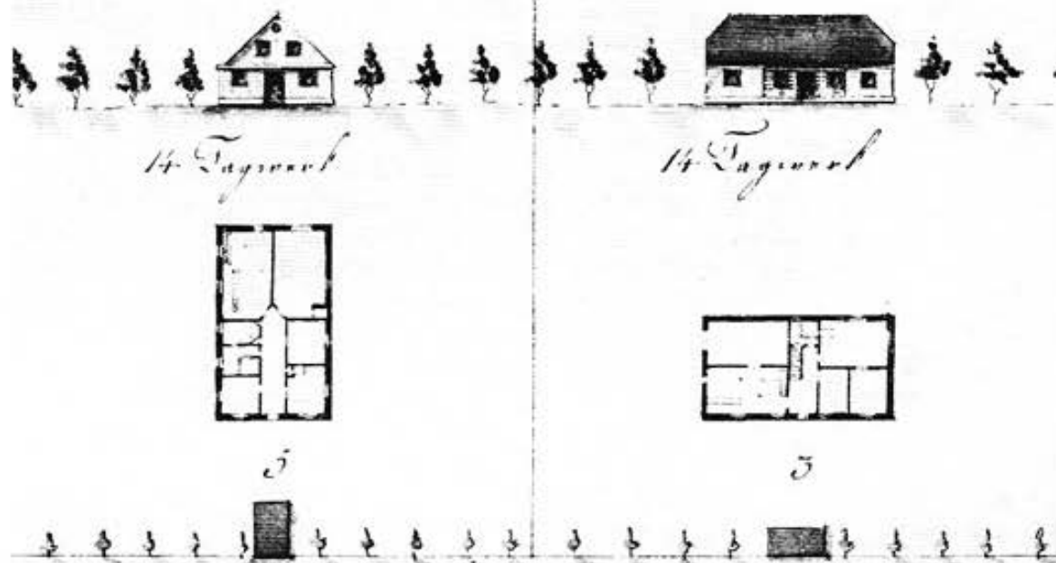
Risse der Musterhäuser in Karlsfeld aus dem Jahre 1802. Bayer. Hauptstaatsarchiv München Abt. I. Plansammlung Nr. 929
