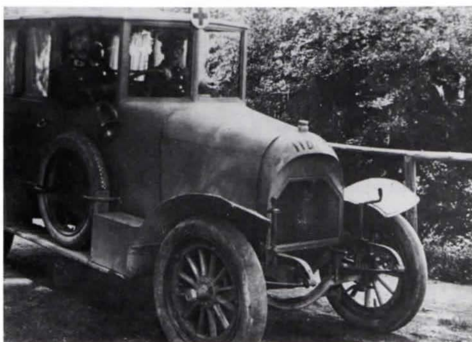
Der zweite »Sanka« der Freiwilligen Sanitätskolonne Dachau. Das gebrauchte Horch-Chassis wurde 1920 vom Roten Kreuz erworben und von Wagnermeister Hans Gessler mit einer bedarfsgerechten Karosserie versehen (Originalaufnahme im Besitz des BRK Dachau).
