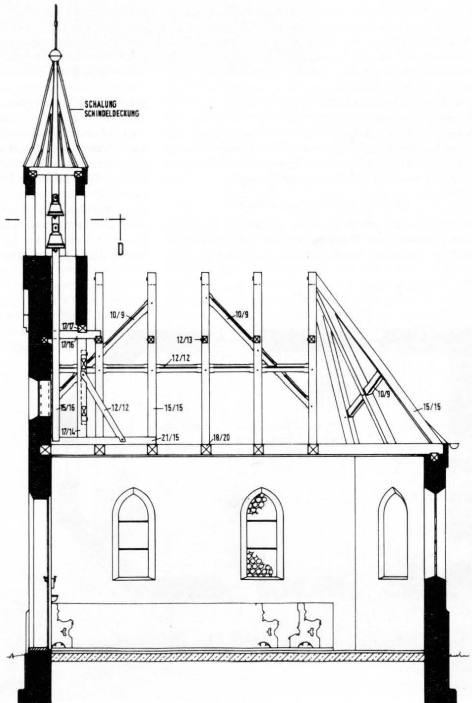
Kapelle St. Maria in Römerthofen, Aufriß. Zeichnung: Architekturbüro Zeh
